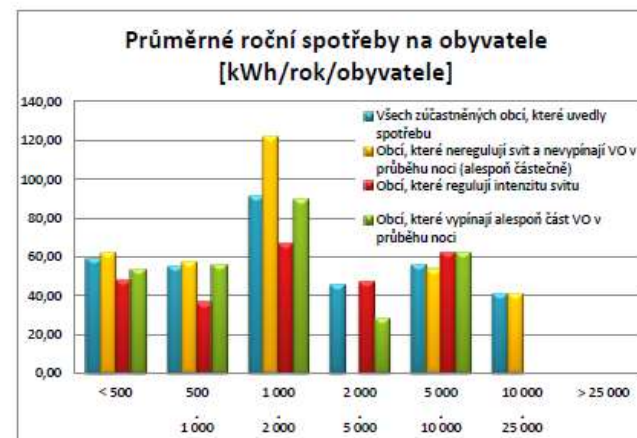
Graf č. 20 – průměrné roční spotřeby elektřiny na obyvatele obcí v rámci jednotlivých kategorií velikostí a způsobu regulace svítu soustavy VO
