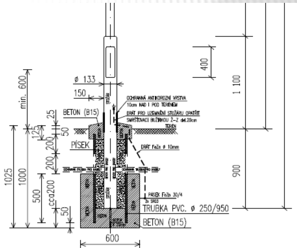
SCHÉMA ZÁKLADU PRO STOŽÁR B6
